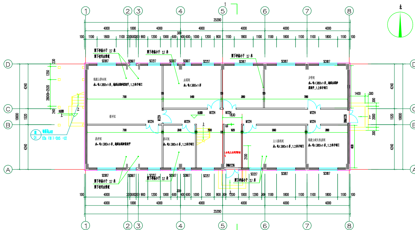
一层平面图 1:100
