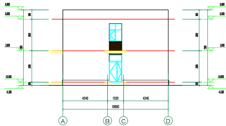
①~③轴立面图1:100
