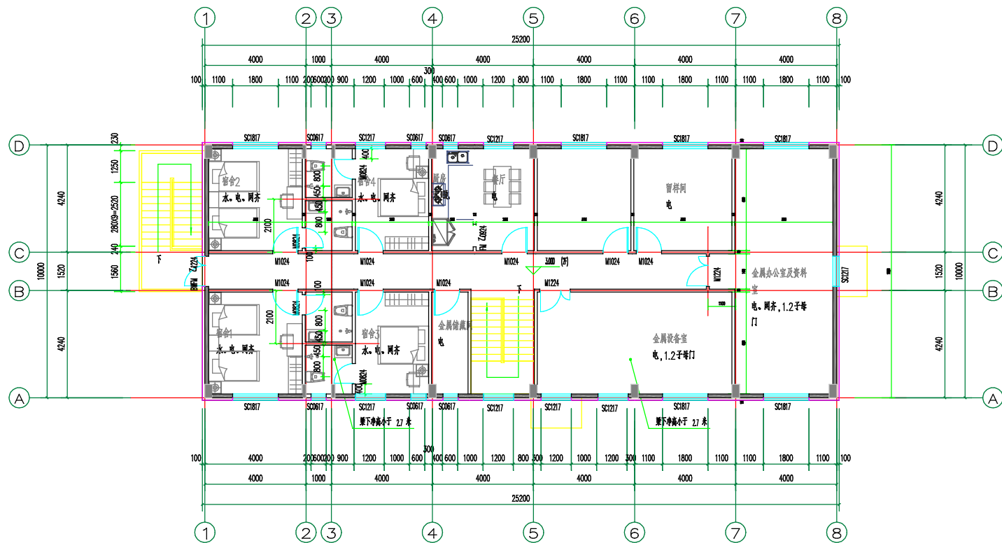
二层平面图 1:100
